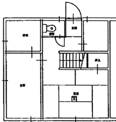
1階平面図
