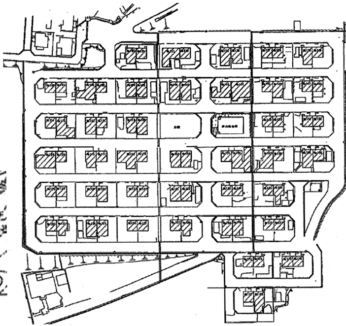
岸山地区 改良住宅 配置図
