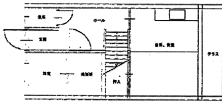
1 階平面図
