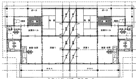
間取り図
