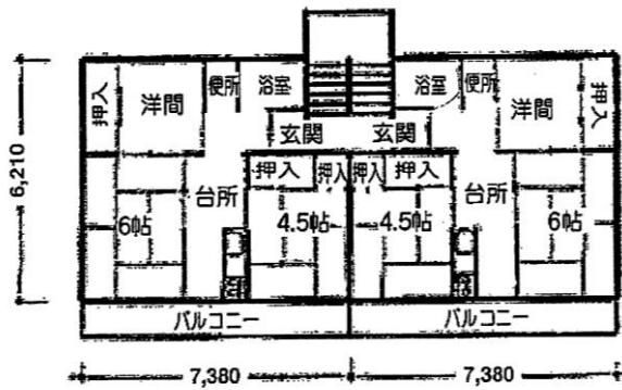
<間取り図(2)>
