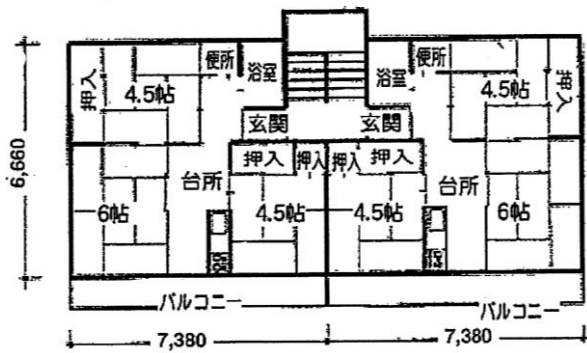
<間取り図(1)>
