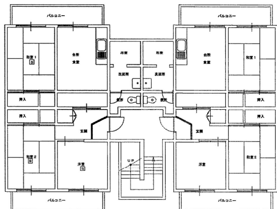
間取り図
